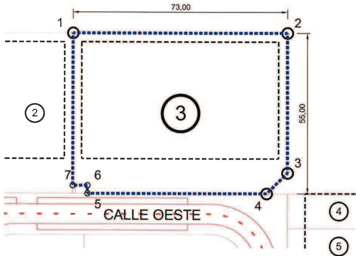
Coordenadas planas referidas a bases del Polígono
